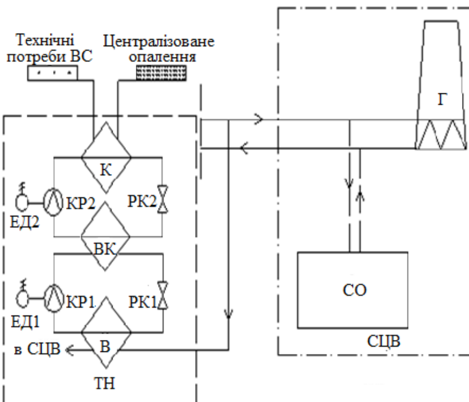
Рис. 3. ТНТ для систем централізованого опалення та технологічних потреб:
