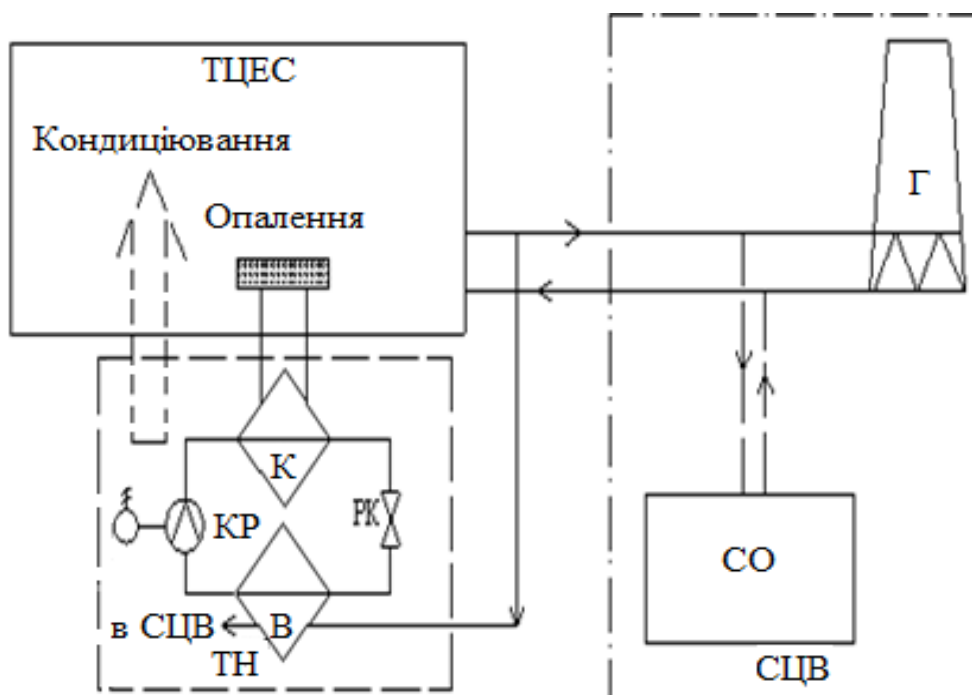
Рис. 2. ТНТ на електростанціях для теплопостачання та кондиціювання: ЕД – електродвигун; КР – компресор; К – конденсатор; РК – терморегулюючий вентиль; В – випарник; ТН – тепловий насос; СЦВ – система циркуляційного водозабезпечення; СО – ставок охолоджувач; Г – градирня
