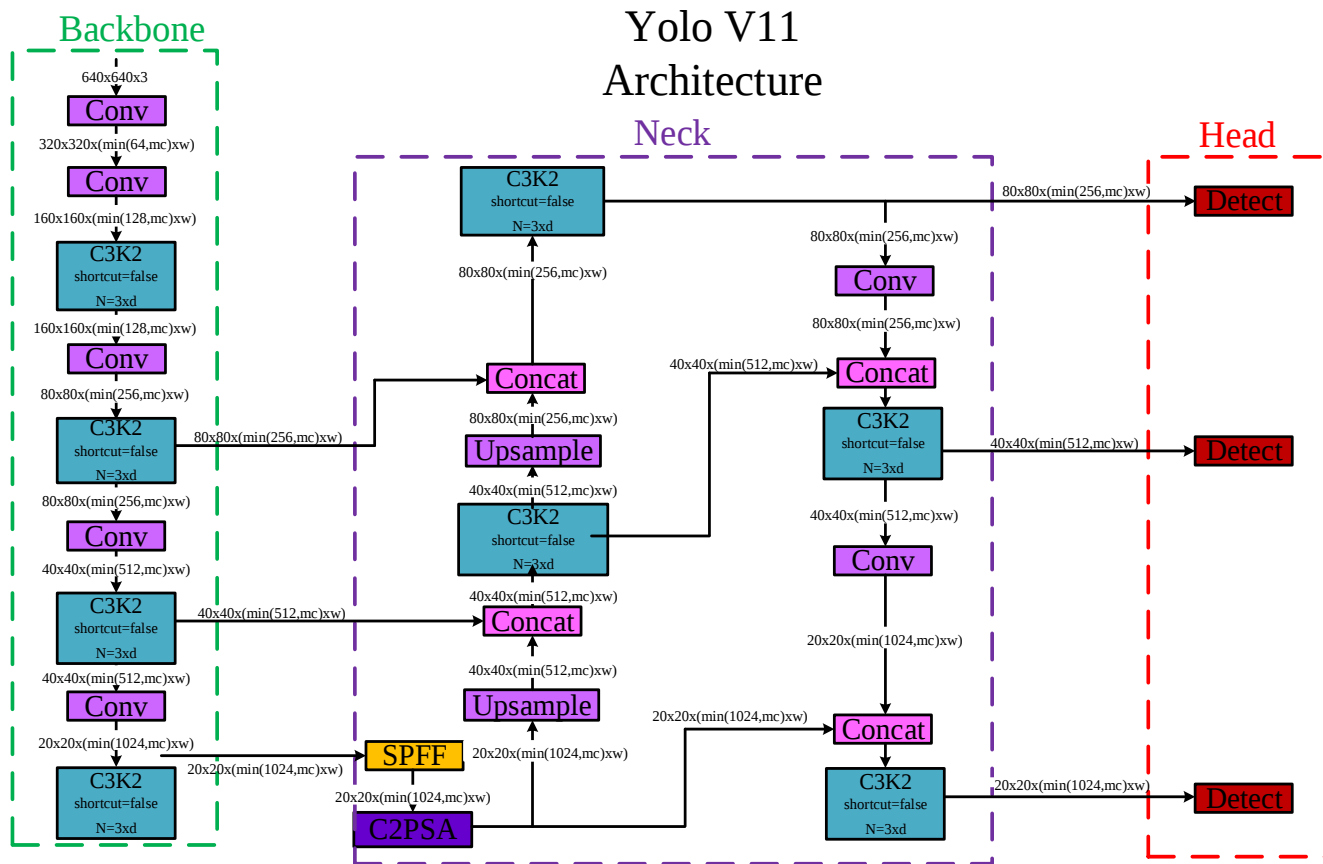
Рис. 2. Структурна схема YOLOv11
