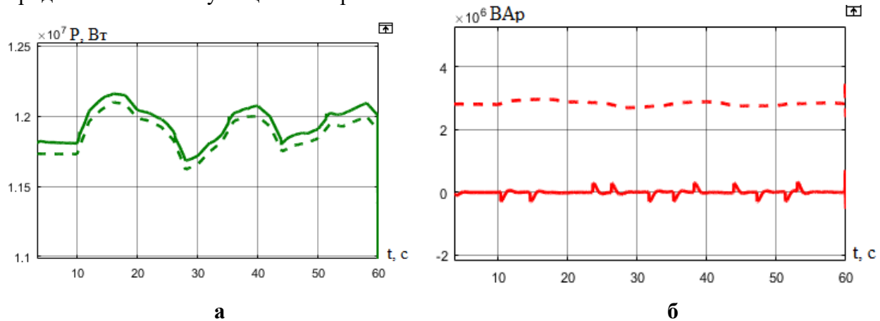
Рис. 4. Рівні споживання активної та реактивної потужності на ввіді системи (штрихова лінія – до використання компенсаційних пристроїв; суцільна лінія – після використання компенсаційних пристроїв):
