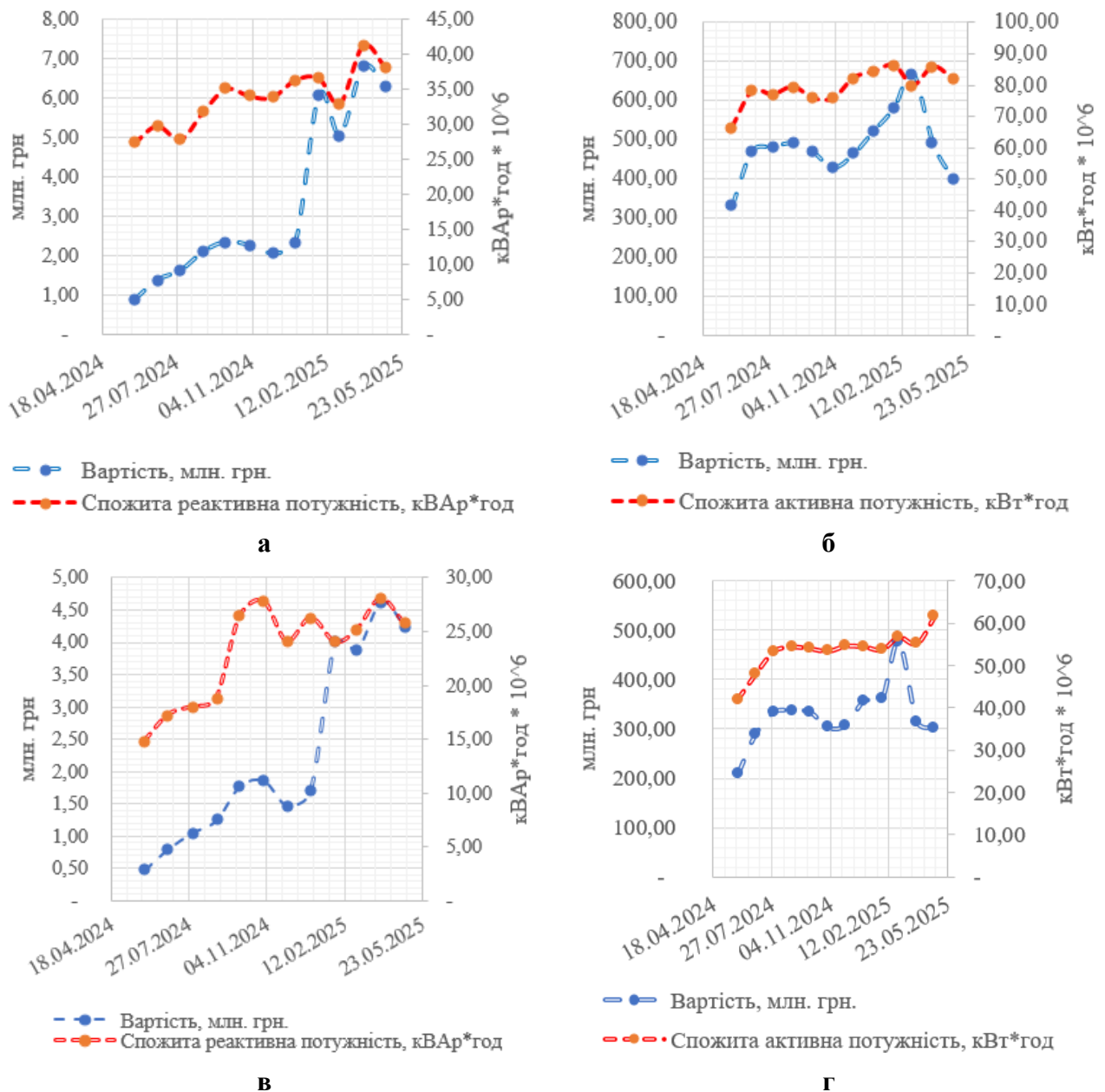
Рис. 1. Споживання електричної енергії гірничозбагачувальними комбінатами за 2024-2025 роки:
